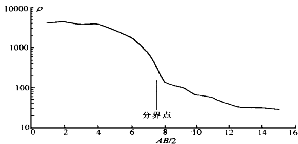
图 3 马庄矿钻孔二极电剖面曲线
