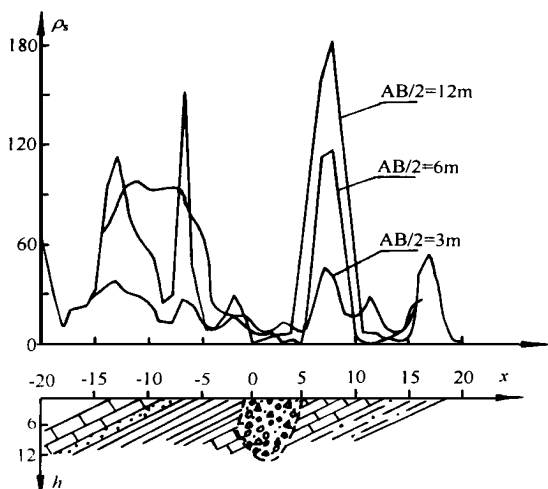
图 2 涟水矿多极距对称四极剖面曲线
