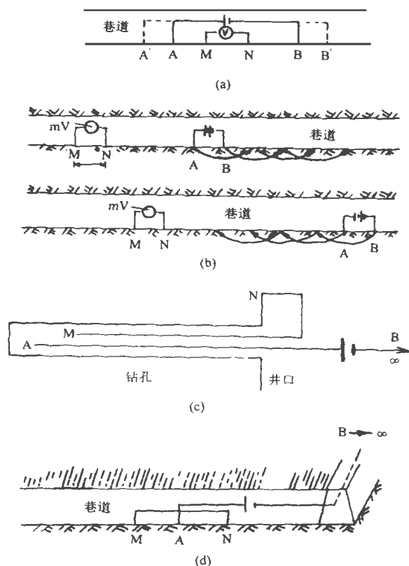
图1 矿井电剖面法工作装置
