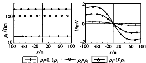
图 5 顶板岩性变化情况(垂向单极-偶极法)
