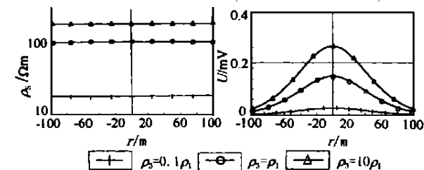
图 5 顶板岩性变化情况(垂向单极-偶极法)
