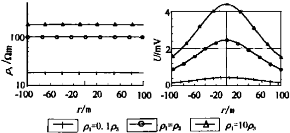
图 3 顶板岩性变化情况(平行单极—偶极法)
