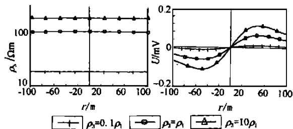
图 7 底板岩性变化情况(垂向偶极-偶极法)
